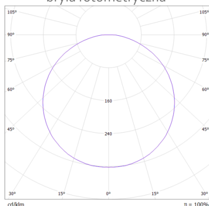
bryła fotometryczna
